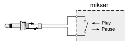
④ Funkcja "fader start" dla przełącznika typu on/off
