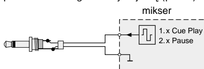
⑥ Funkcja "fader start" z wykorzystaniem impulsowego sygnału sterującego.
