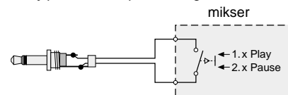
⑤ Regulacja startu i pauzy za pomocą włącznika monostabilnego
