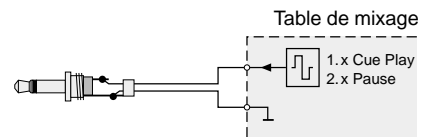
⑥ Démarrage électrique par impulsion de commande
